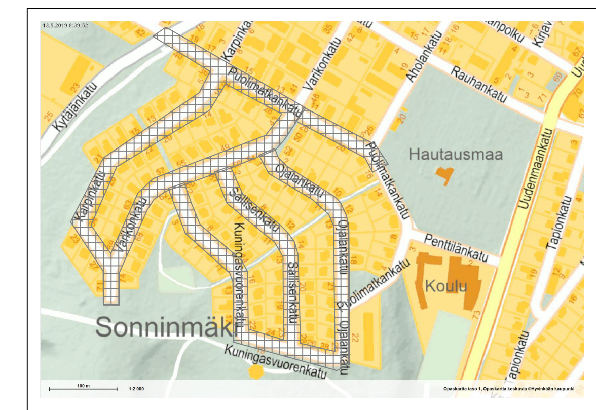
OSOITEKARTTA
